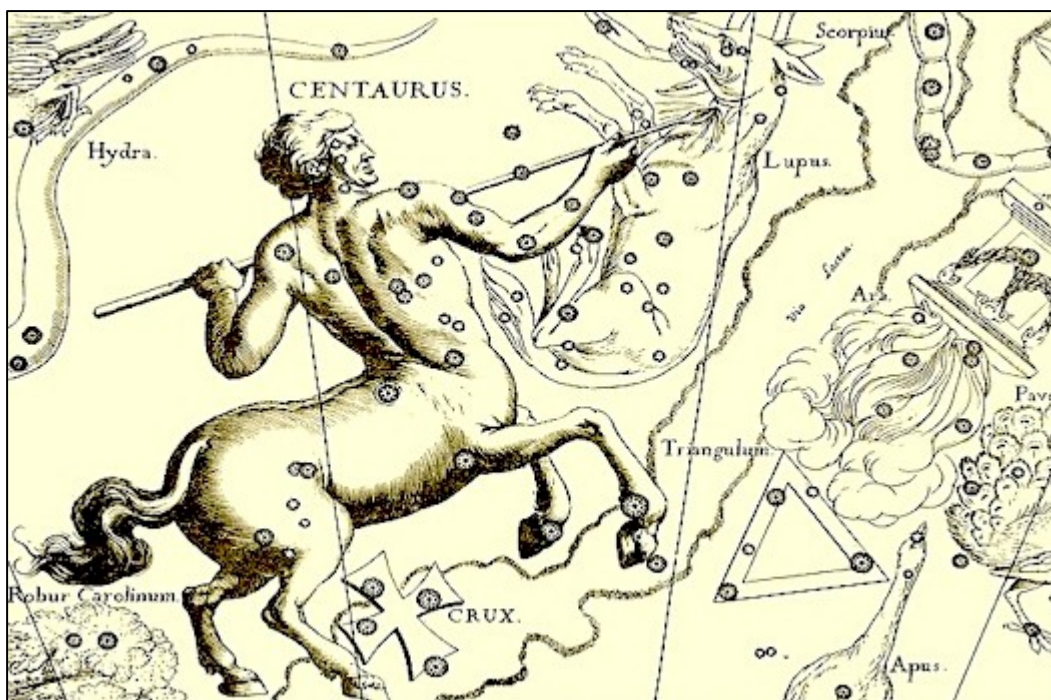
Hevelius, Firmamentum , 1690
